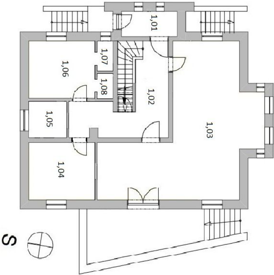
PŮDORYS PŘÍZEMÍ
